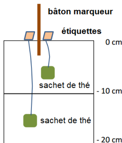
Figure 1 : Analyse de la décomposition dans deux couches de sol
